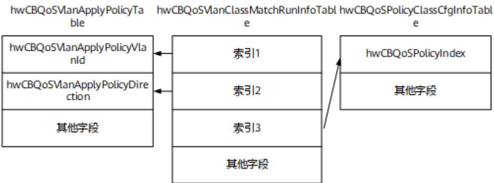
图 23-6 流分类规则统计信息表与 VLAN 流策略表的表间关系
