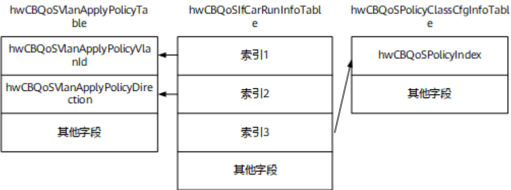
图 23-7 CAR 统计信息表与 VLAN 流策略表的表间关系
