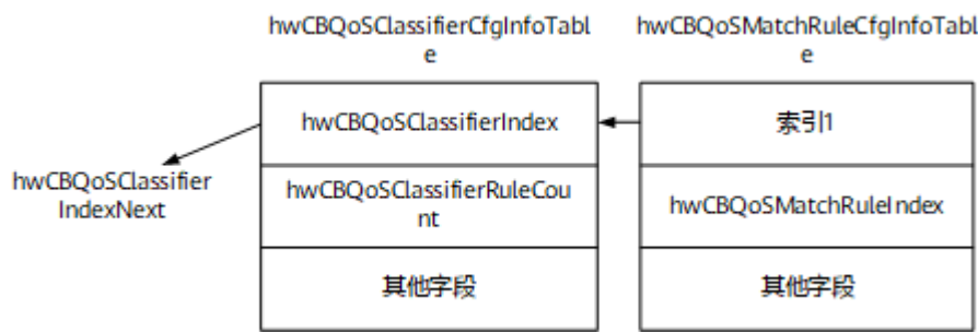
图 23-1 基于规则的流分类配置表的表间关系
